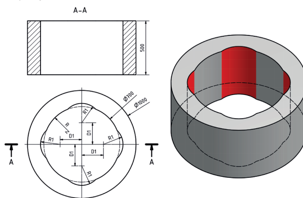
Mazací kapsy u kluzného ložiska, vyrobeno soustružením
